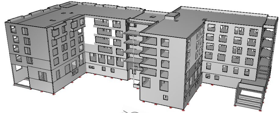
3D FEM Rechenmodell Infograph - Bethanien
